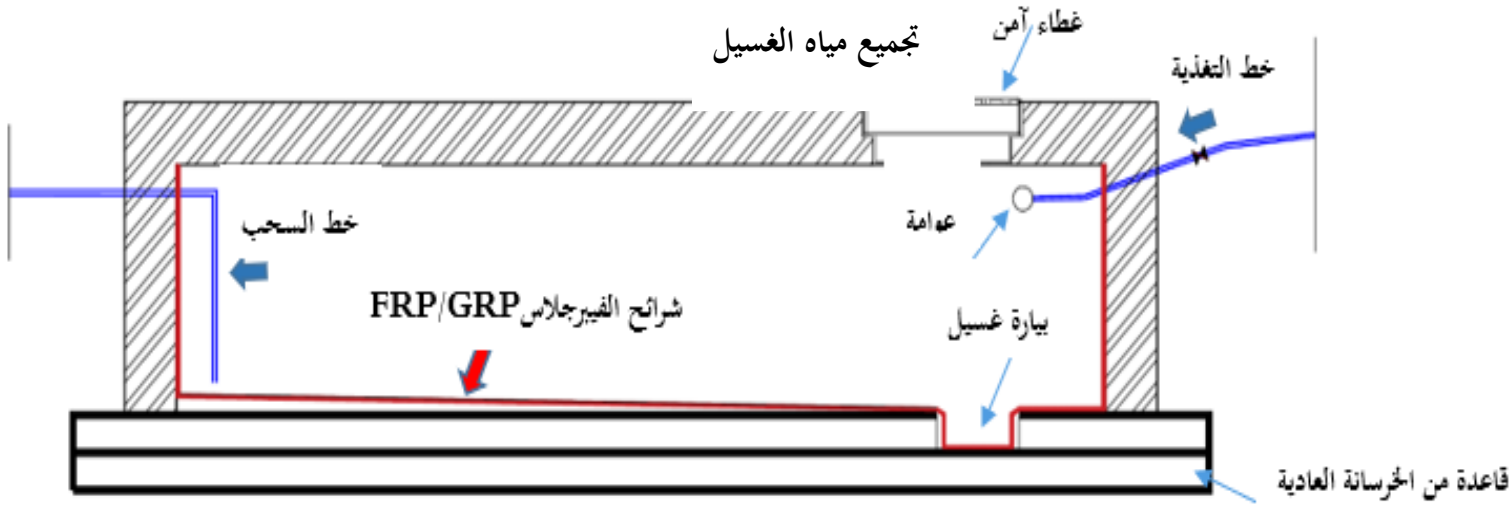
عزل الجدران الداخلية للخرسانة بشرايح الفايبر جلاس FRP/GRP
