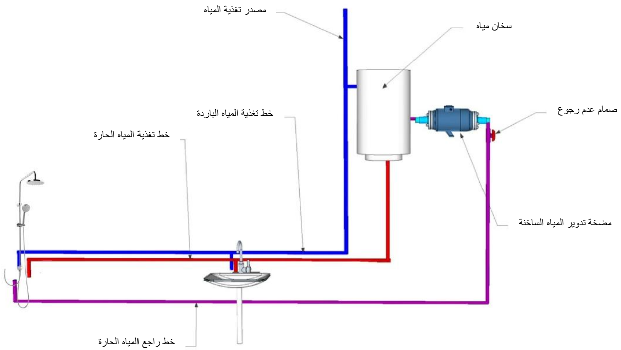
شكل 3 : نموذج للدائرة المغلقة بين سخان المياه والصنابير
