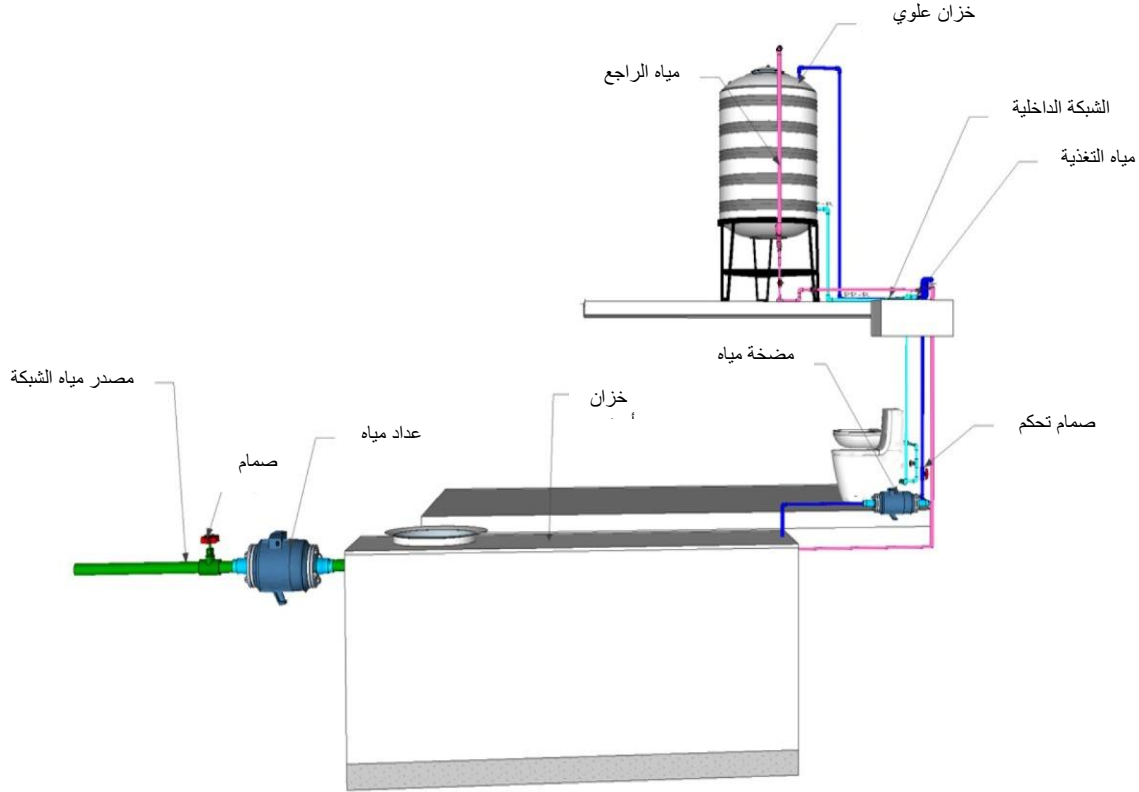
شكل 2: رسم الدائرة المغلقة بين الخزان الأرضي والعلوي
