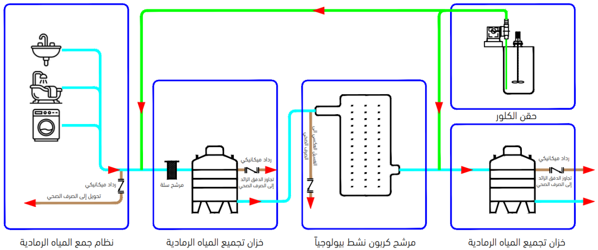
الشكل 5: المرشحات الميكانيكية (لاستخدام الماء في غسل المراحيض) - مرشح الكربون المنشط بيولوجيا
